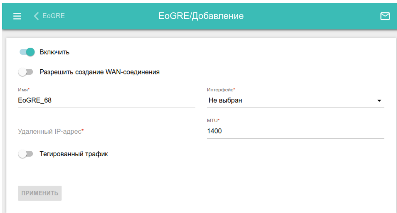
Рисунок 120. Страница добавления EoGRE-туннеля.
