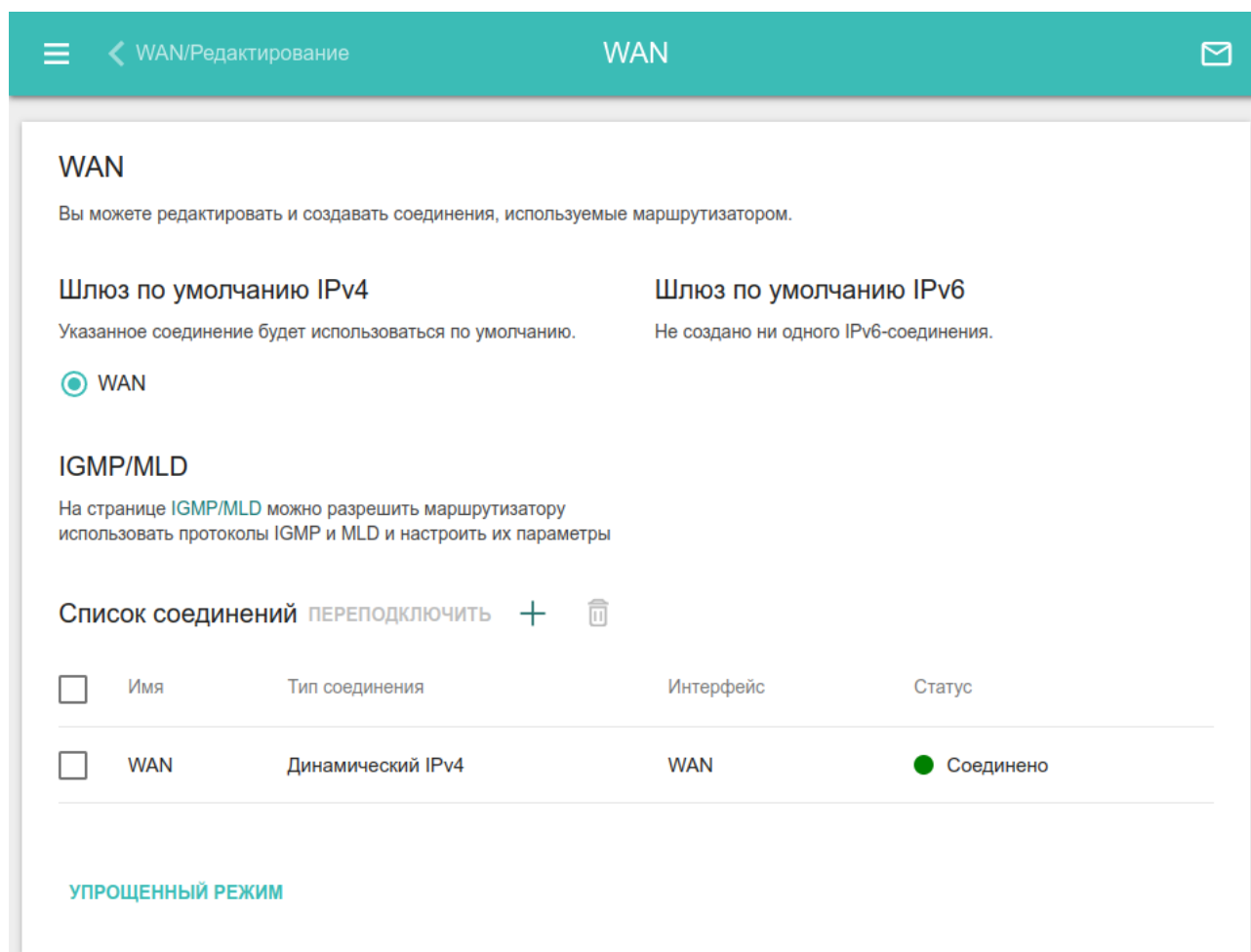
Рисунок 55. Страница Настройка соединений / WAN . Расширенный режим.
