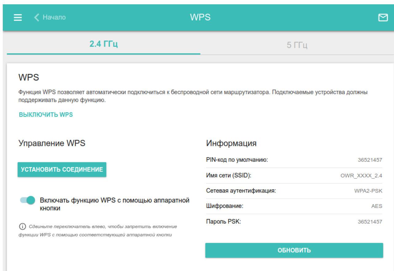
Рисунок 116. Страница для настройки функции WPS.
