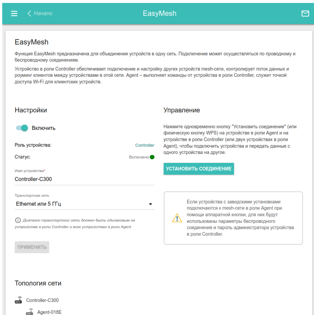
Рисунок 123. Страница Wi-Fi / EasyMesh.
