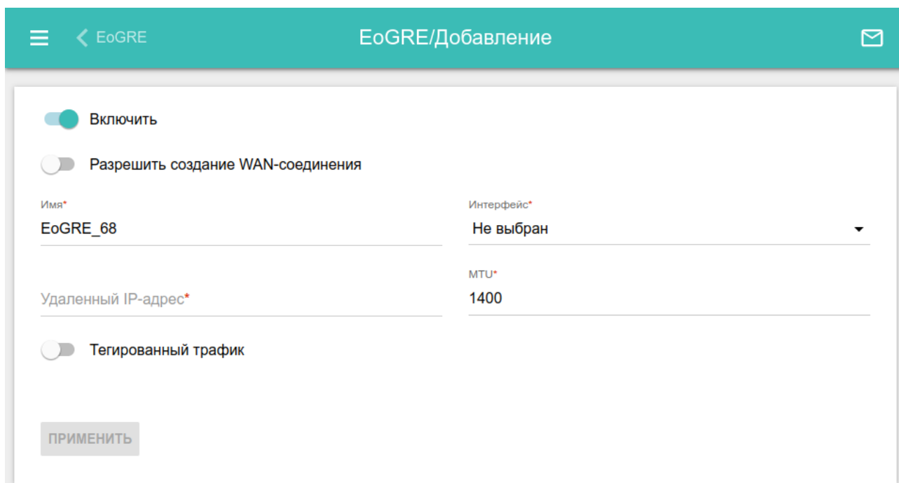
Рисунок 109. Страница добавления EoGRE-туннеля.
