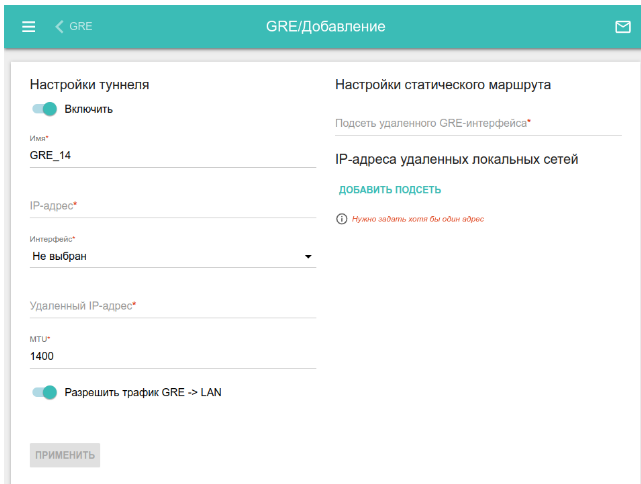
Рисунок 100. Страница добавления GRE-туннеля.
