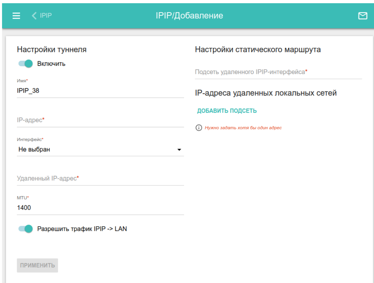
Рисунок 102. Страница добавления IPIP-туннеля.
