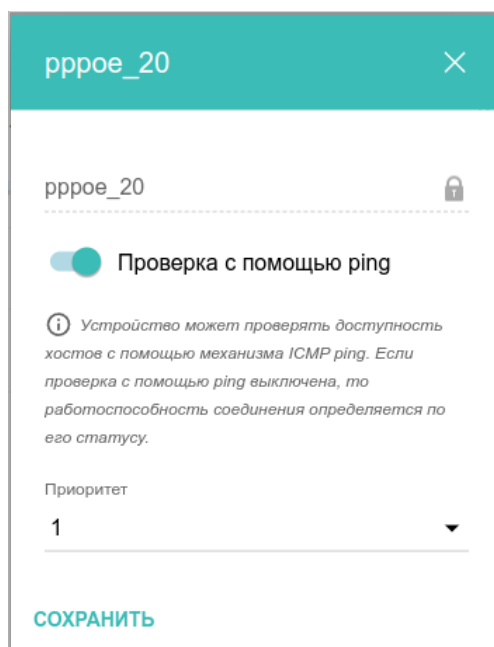
Рисунок 92. Окно изменения уровня приоритета соединения.
