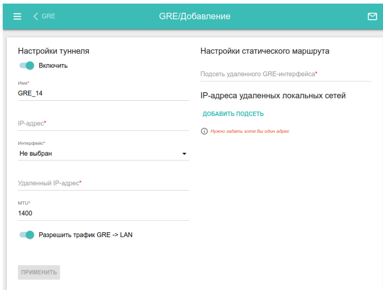
Рисунок 95. Страница добавления GRE-туннеля.
