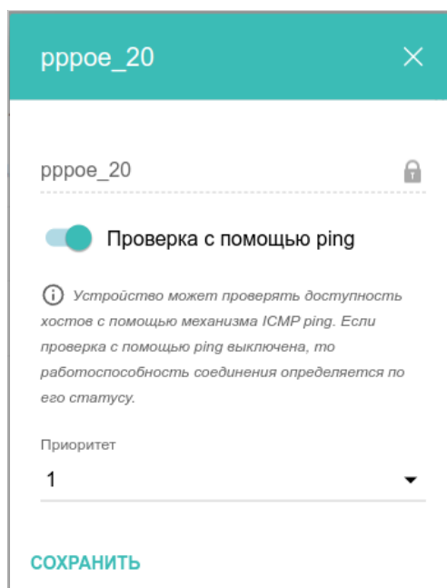
Рисунок 88. Окно изменения уровня приоритета соединения.
