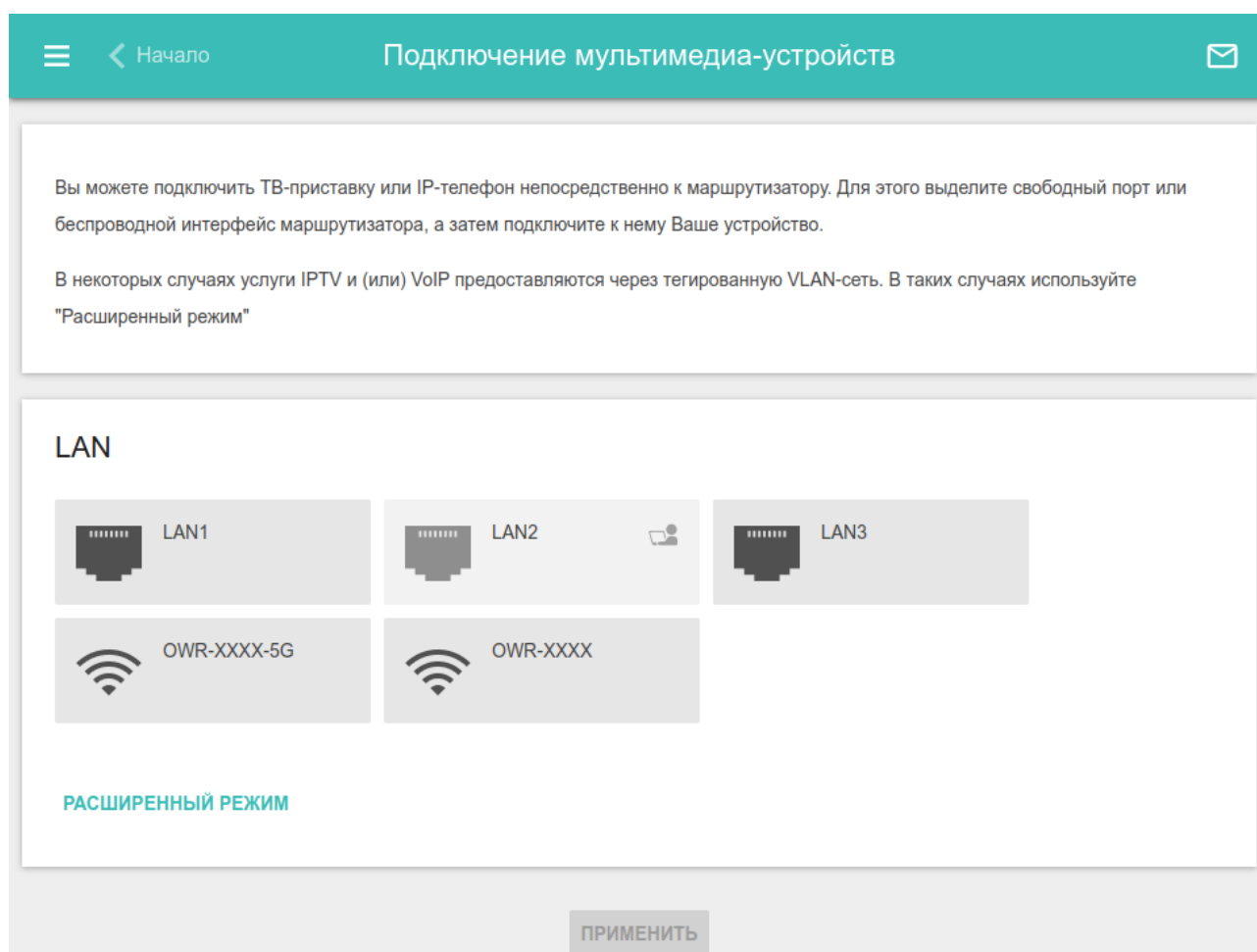
Рисунок 42. Мастер подключения мультимедиа-устройств. Упрощенный режим.
