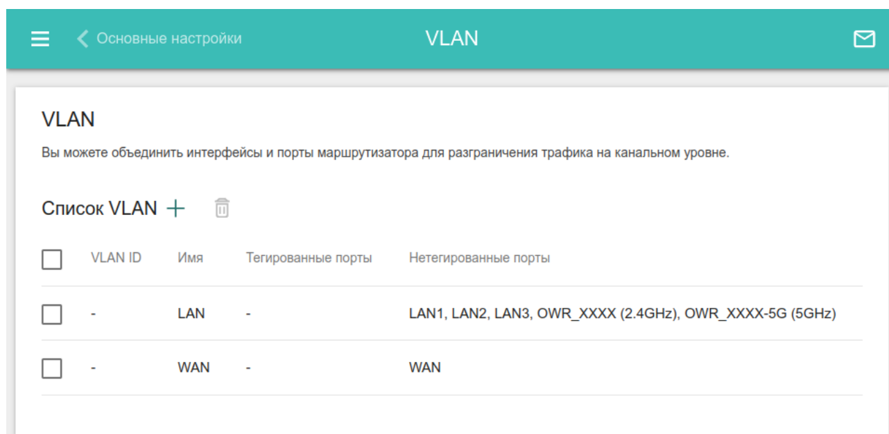
Рисунок 99. Страница Дополнительно / VLAN .
