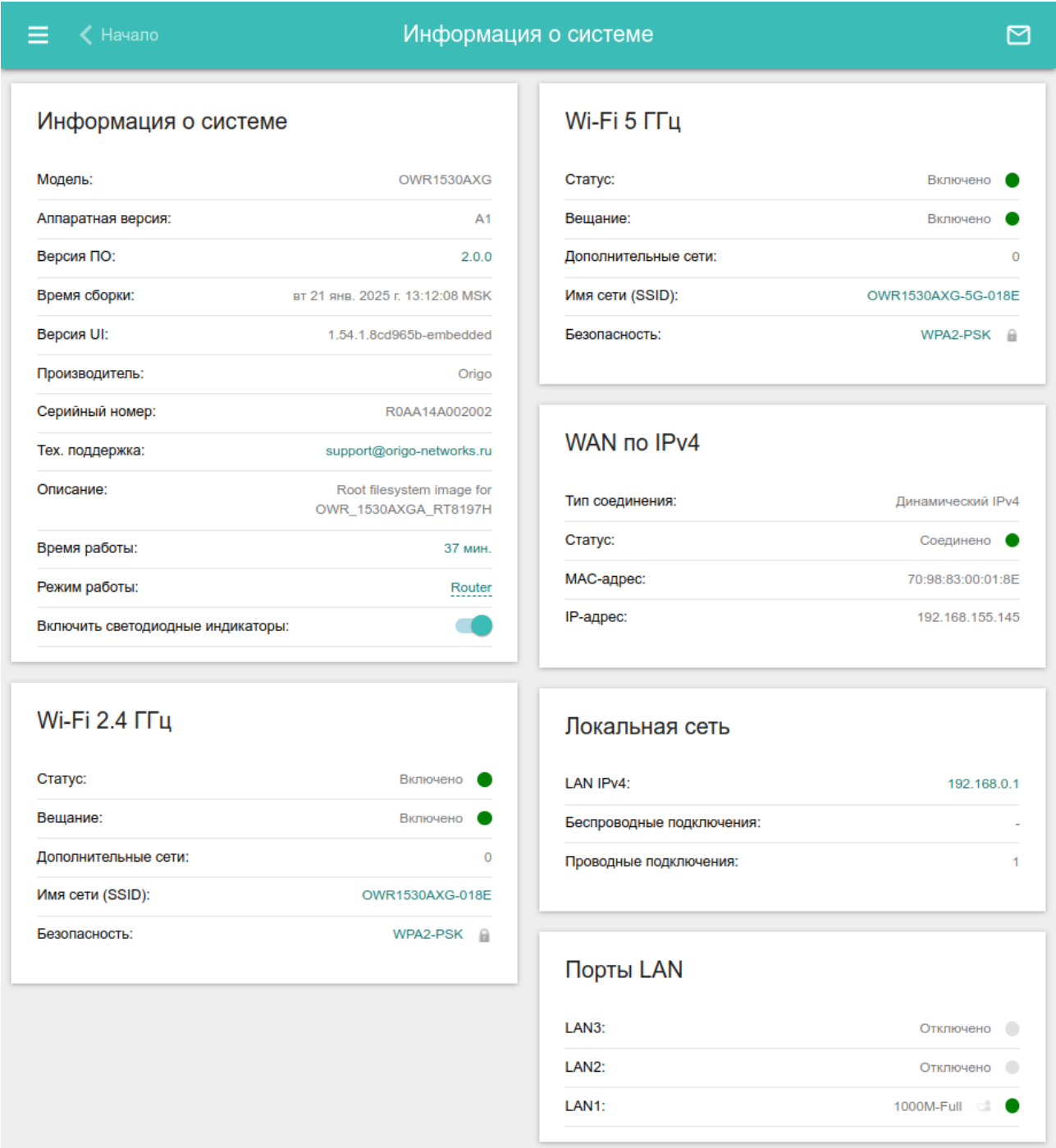
Рисунок 12. Страница информации о системе.
