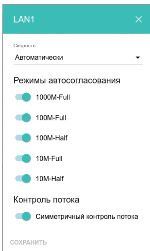
Рисунок 105. Окно изменения настроек порта маршрутизатора.
