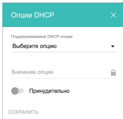
Рисунок 77. Настройка локального интерфейса. Вкладка IPv4. Окно для настройки опции DHCP.
