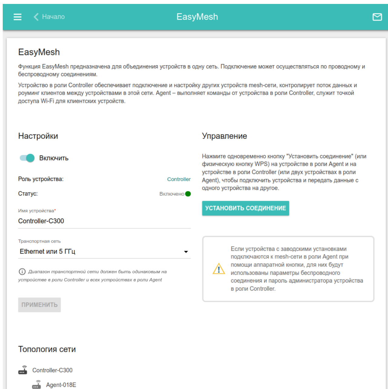
Рисунок 97. Страница Wi-Fi / EasyMesh .
