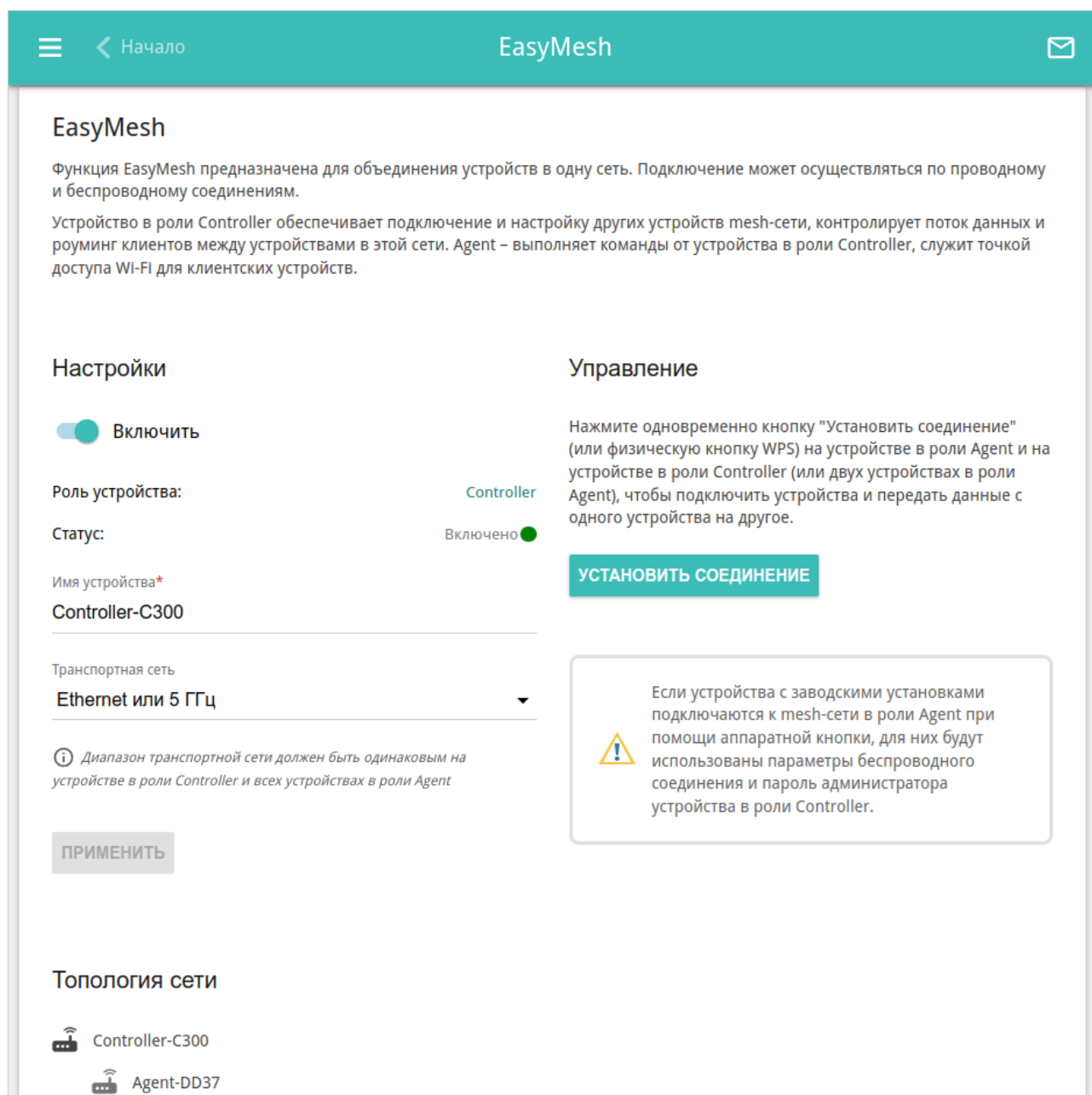
Рисунок 126. Страница Wi-Fi / EasyMesh .
