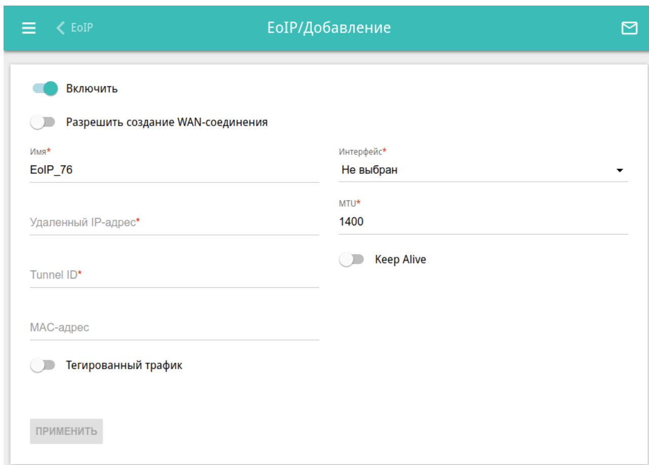
Рисунок 112. Страница добавления EoIP-туннеля.
