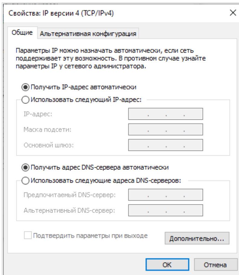
Рисунок 5. Окно свойств протокола TCP/IPv4.
