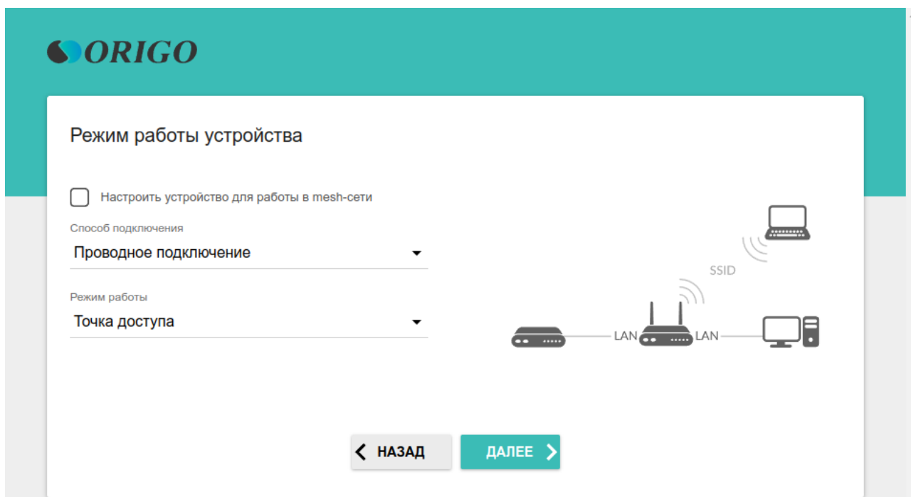
Рисунок 23. Выбор режима работы устройства. Режим Точка доступа .
