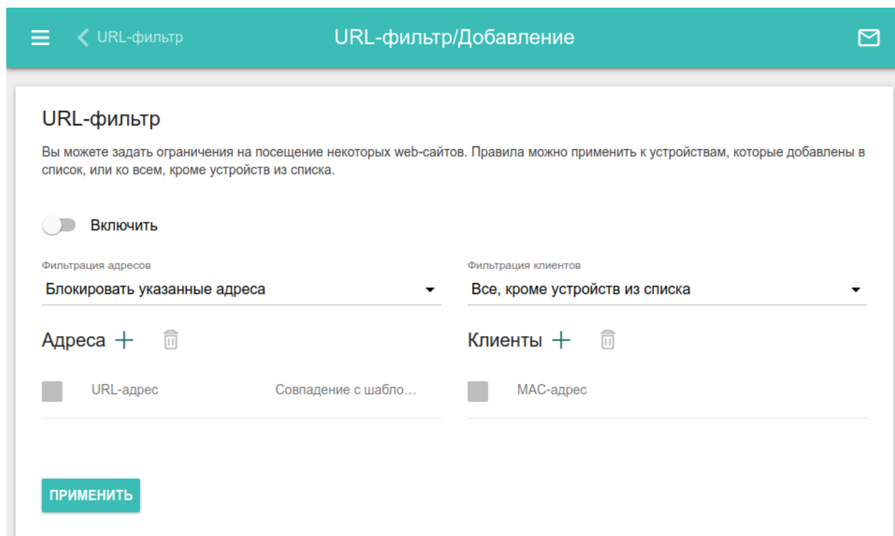
Рисунок 162. Страница добавления правила для URL-фильтра.
