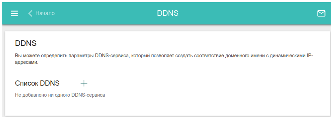
Рисунок 134. Страница Дополнительно / DDNS .
