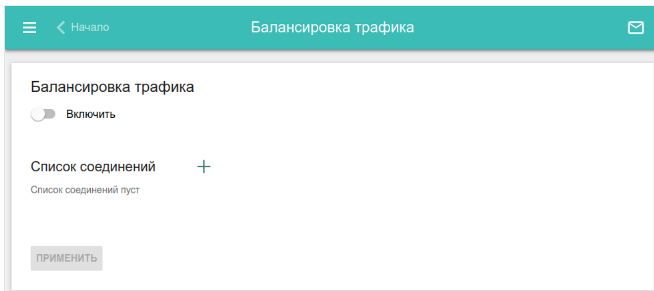
Рисунок 94. Страница Настройка соединений / Балансировка трафика .
