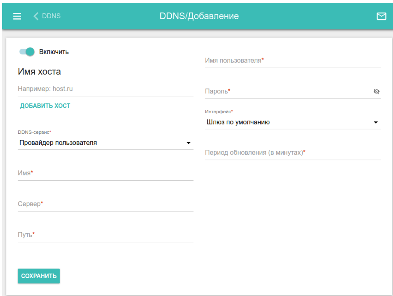
Рисунок 135. Страница добавления нового DDNS-сервиса.
