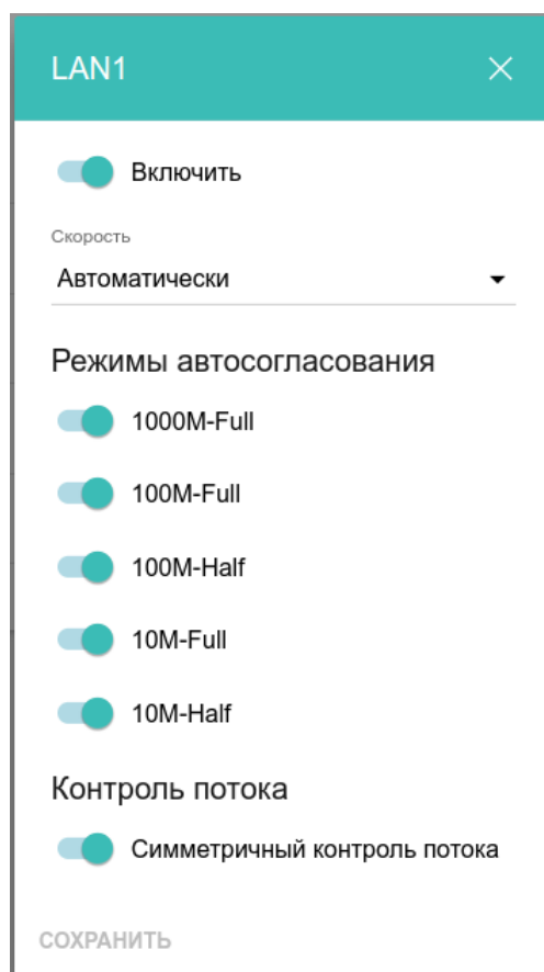
Рисунок 137. Окно изменения настроек порта маршрутизатора.
