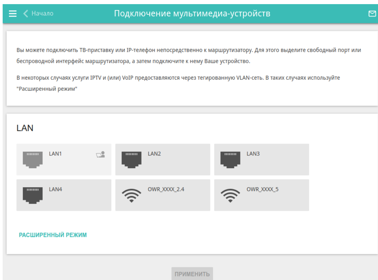
Рисунок 43. Мастер подключения мультимедиа-устройств. Упрощенный режим.
