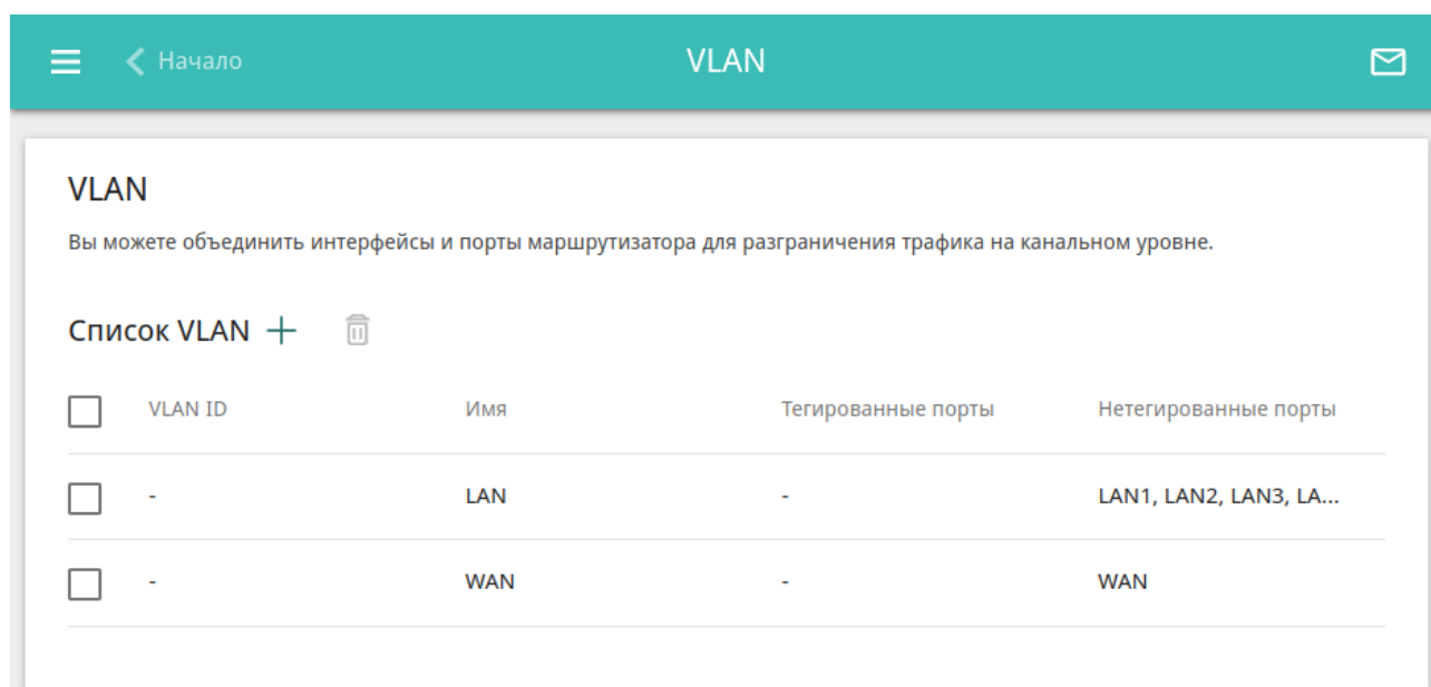
Рисунок 128. Страница Дополнительно / VLAN .
