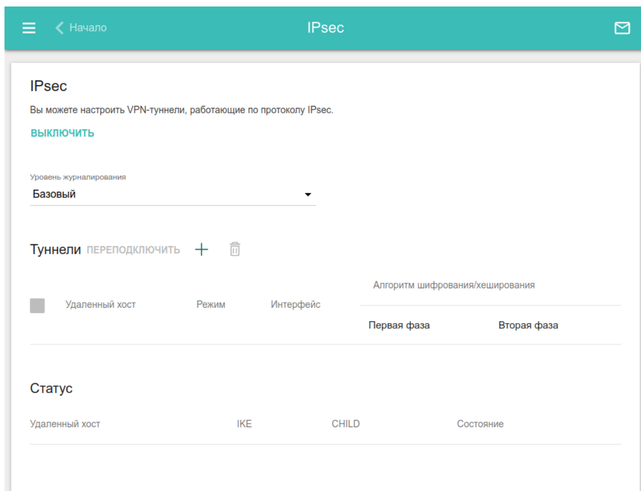
Рисунок 96. Страница VPN / IPsec .
