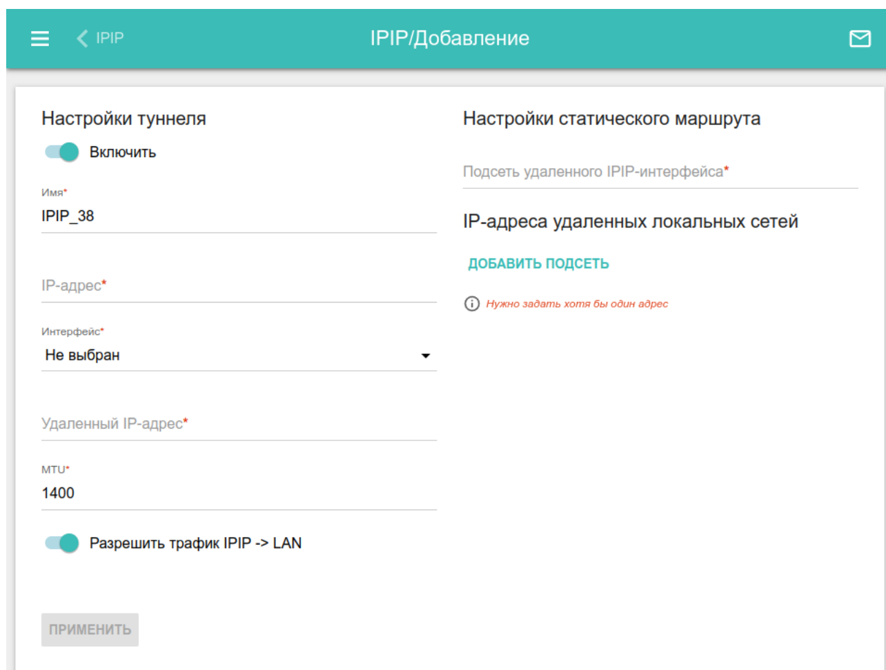
Рисунок 103. Страница добавления IPIP-туннеля.
