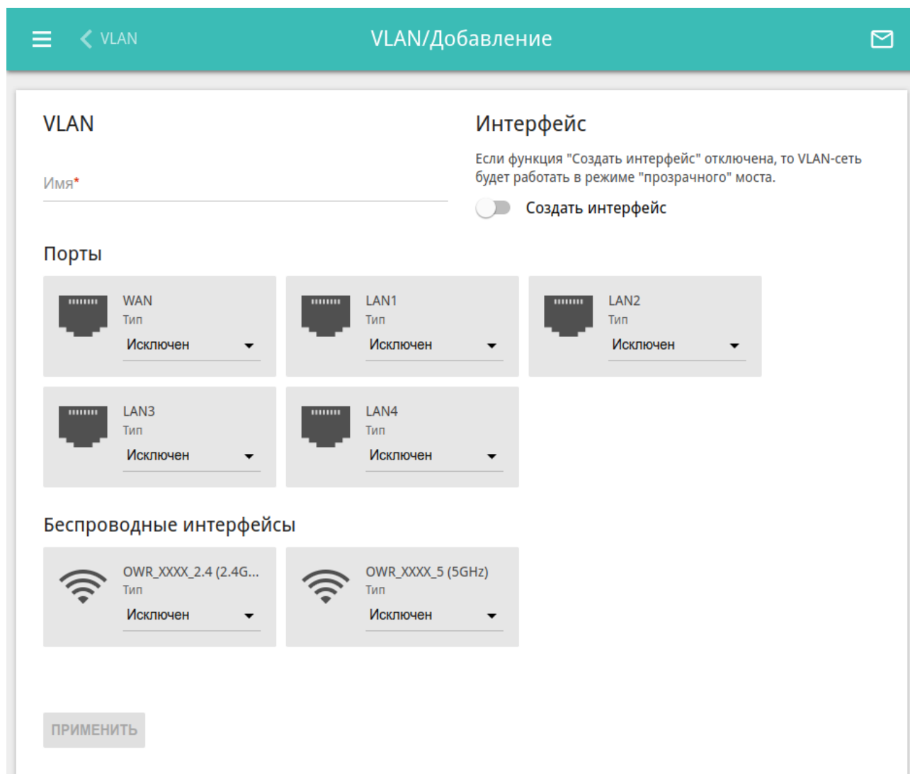
Рисунок 125. Страница добавления VLAN-сети.
