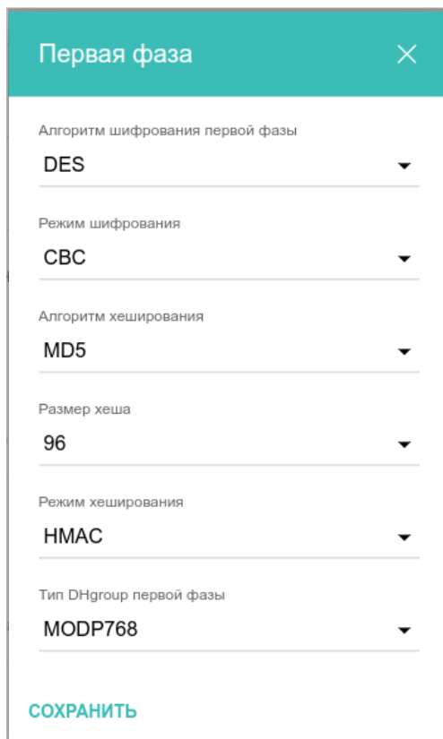
Рисунок 96. Окно настройки первой фазы IPsec-туннеля. Раздел Первая фаза .
