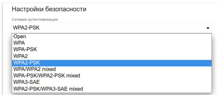
Рисунок 113. Типы аутентификации, поддерживаемые маршрутизатором.
