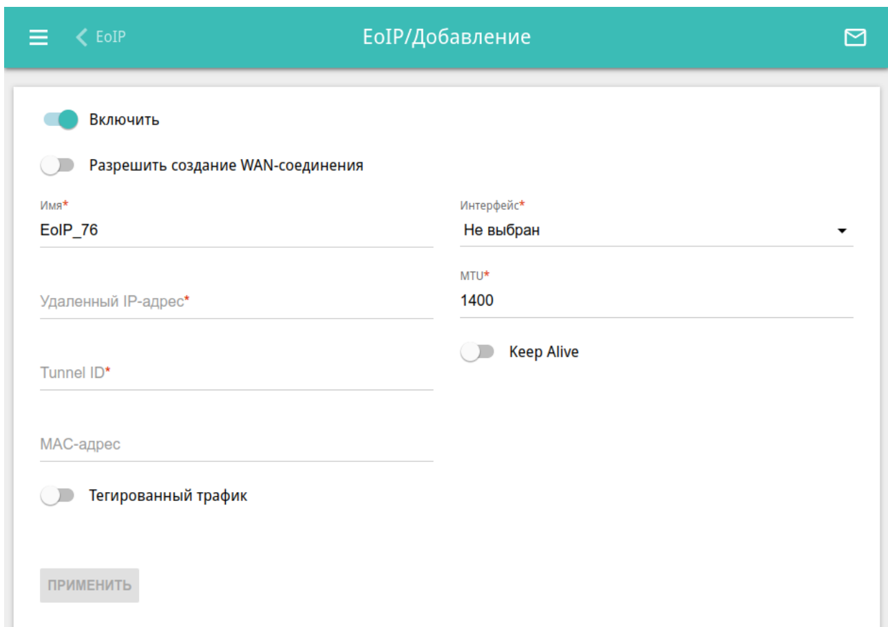
Рисунок 110. Страница добавления EoIP-туннеля.
