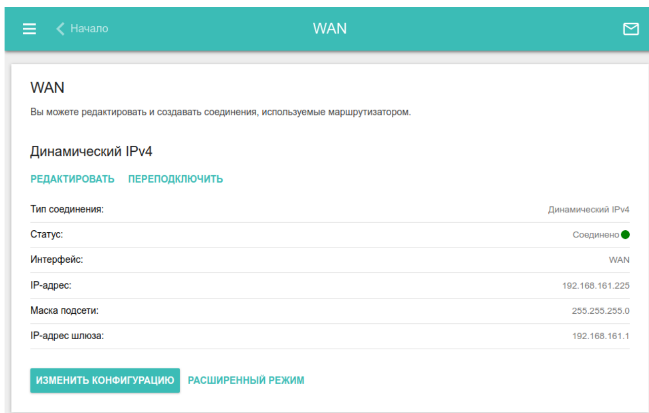
Рисунок 52. Страница Настройка соединений / WAN . Упрощенный режим.
