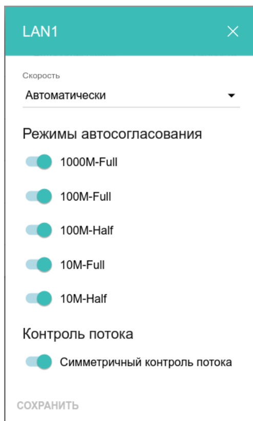
Рисунок 132. Окно изменения настроек порта маршрутизатора.
