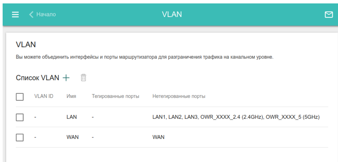
Рисунок 123. Страница Дополнительно / VLAN .
