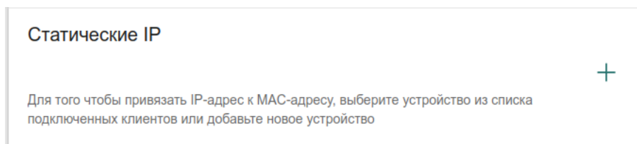
Рисунок 83. Настройка локального интерфейса. Вкладка IPv4 . Раздел для создания связок MAC-IPv4.
