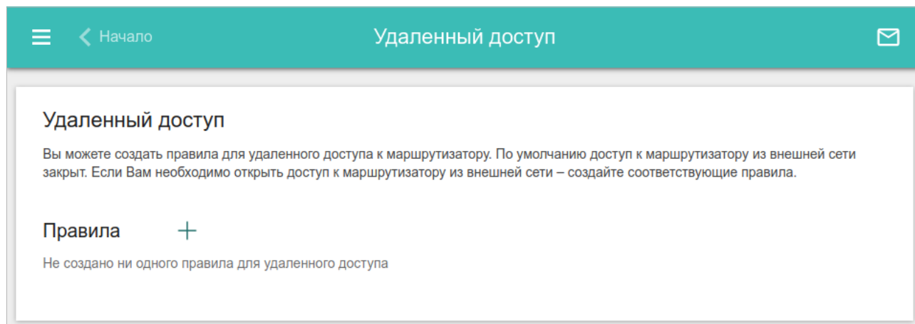
Рисунок 159. Страница Межсетевой экран / Удаленный доступ .
