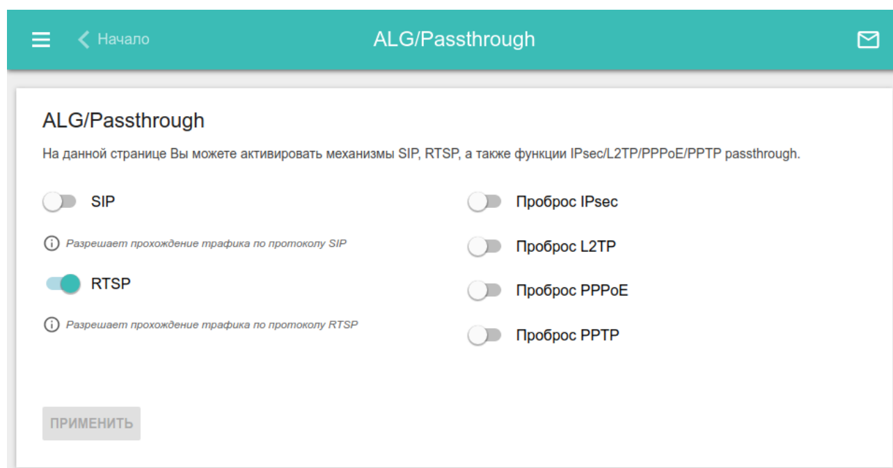
Рисунок 142. Страница Дополнительно / ALG/Passthrough .
