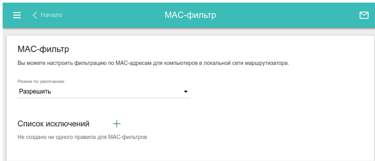
Рисунок 154. Страница Межсетевой экран / MAC-фильтр .
